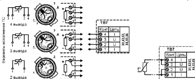
Рис. 4.2 - Варианты подключения ТС
