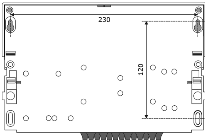
Рис. 4.1 – Схема крепления корпуса ТВ7
