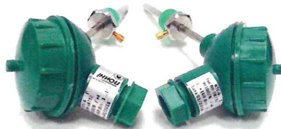
в) Комплект термопреобразователей сопротивления платиновых КТС-Б
