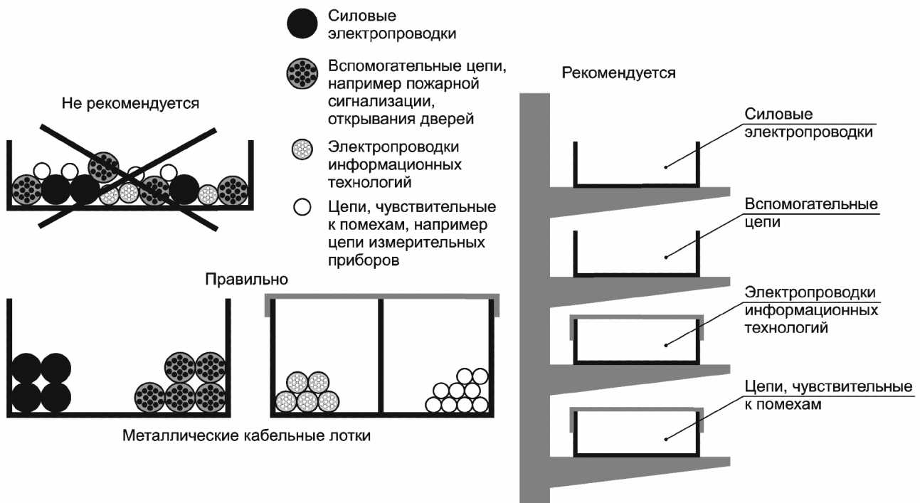
Рисунок 44.R18 — Разделение кабелей в электропроводках
