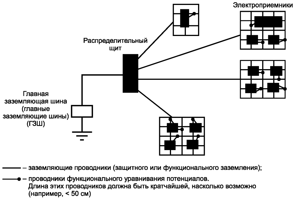
Рисунок 44.R14 — Пример радиального соединения нескольких сетчатых систем
