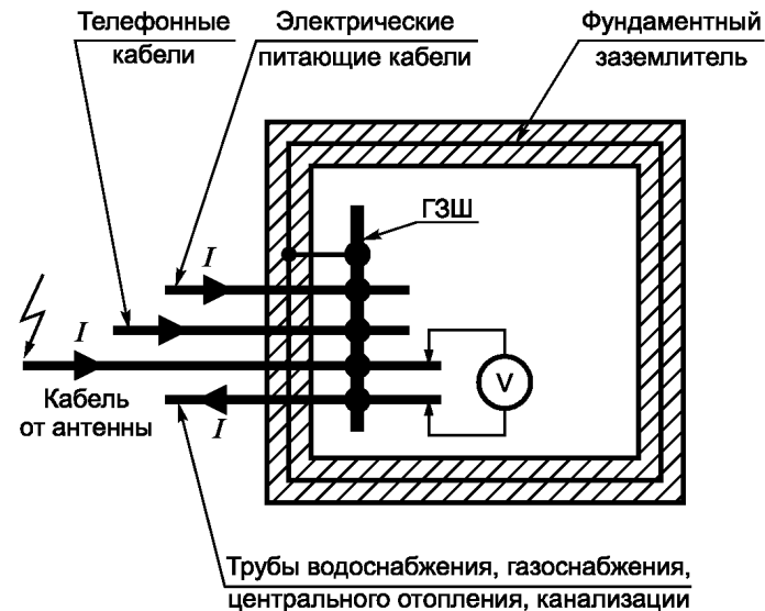
ГЗШ — главная заземляющая шина; I — наведенный ток
