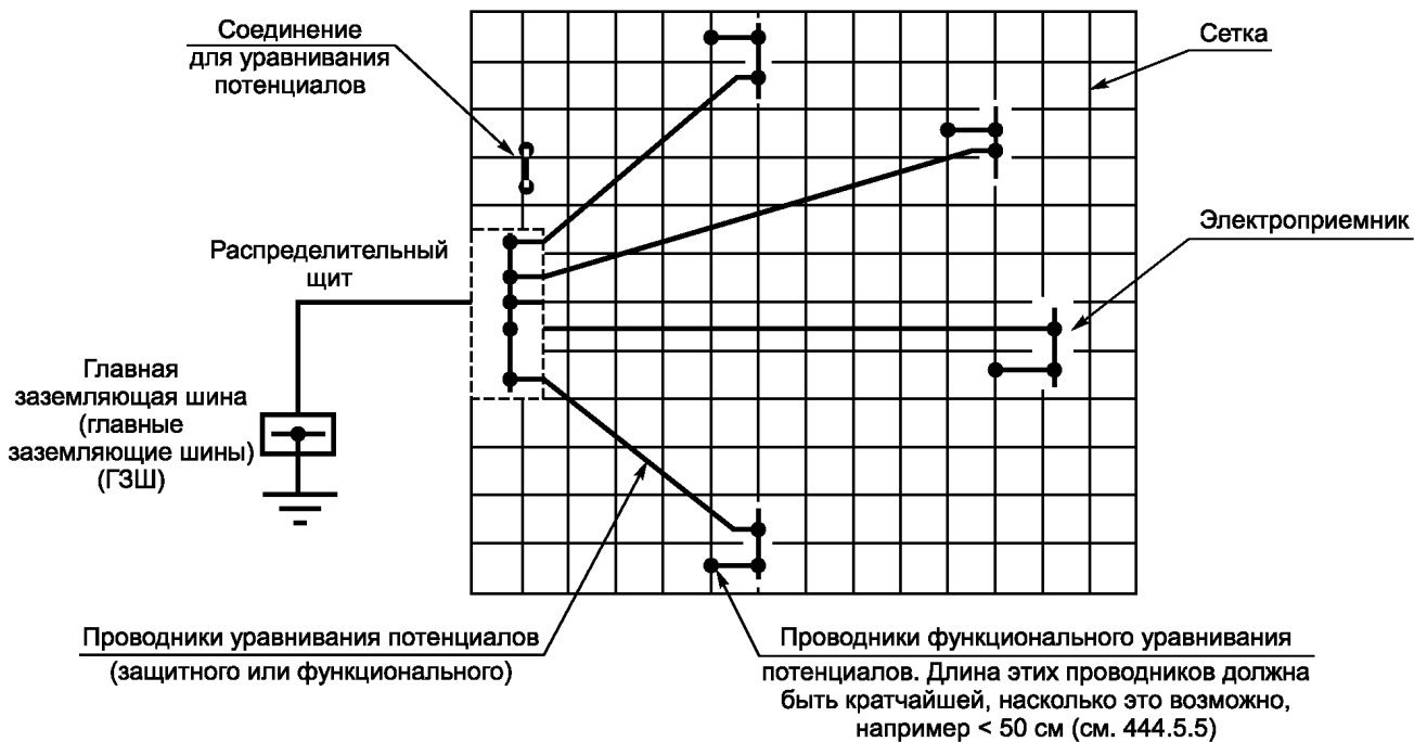
Рисунок 44.R15 — Пример совмещенной сетчато-радиальной системы уравнивания потенциалов
