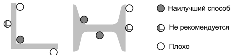
Рисунок 44.R21 — Расположение кабелей внутри элементов металлических конструкций
